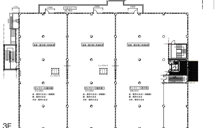
BankART Studio NYK 改修図面 (みかんぐみ)
